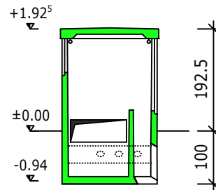
SCHNITT B-B
