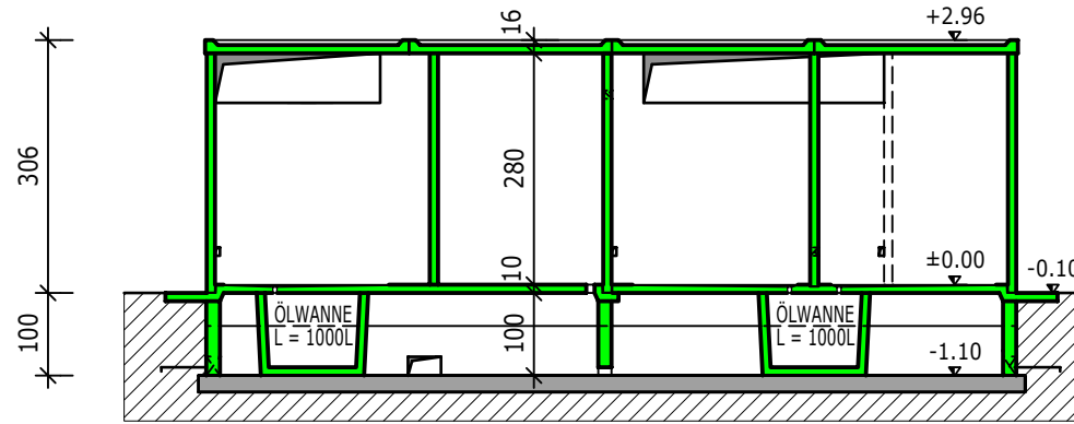
SCHNITT A-A
