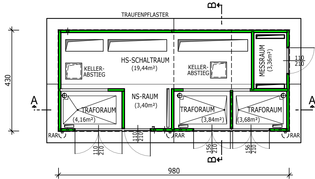
GRUNDRISS
