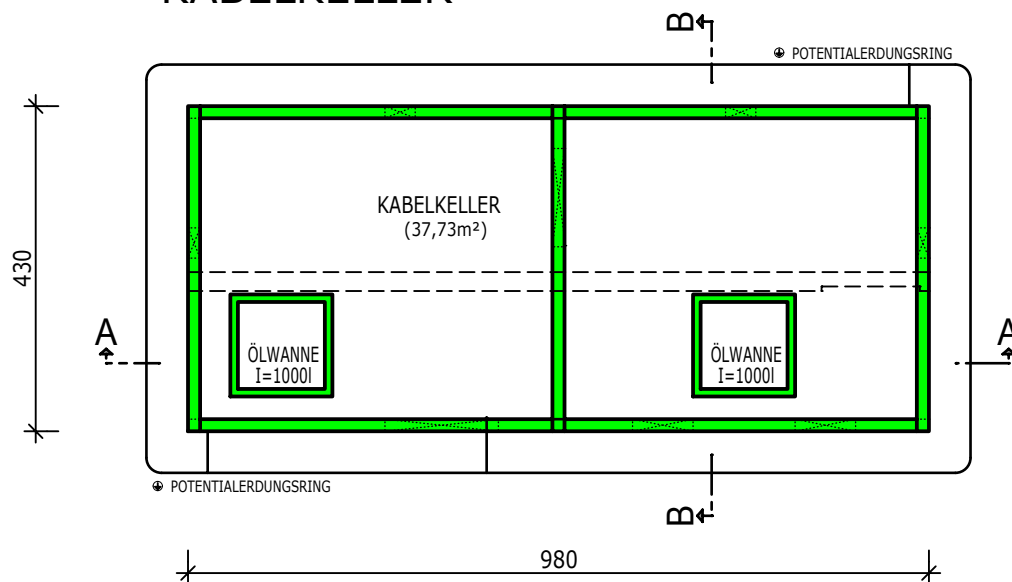
KABELKELLER
