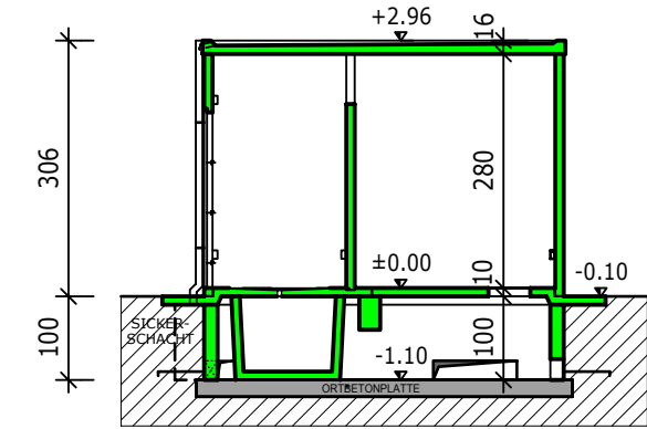
SCHNITT B-B
