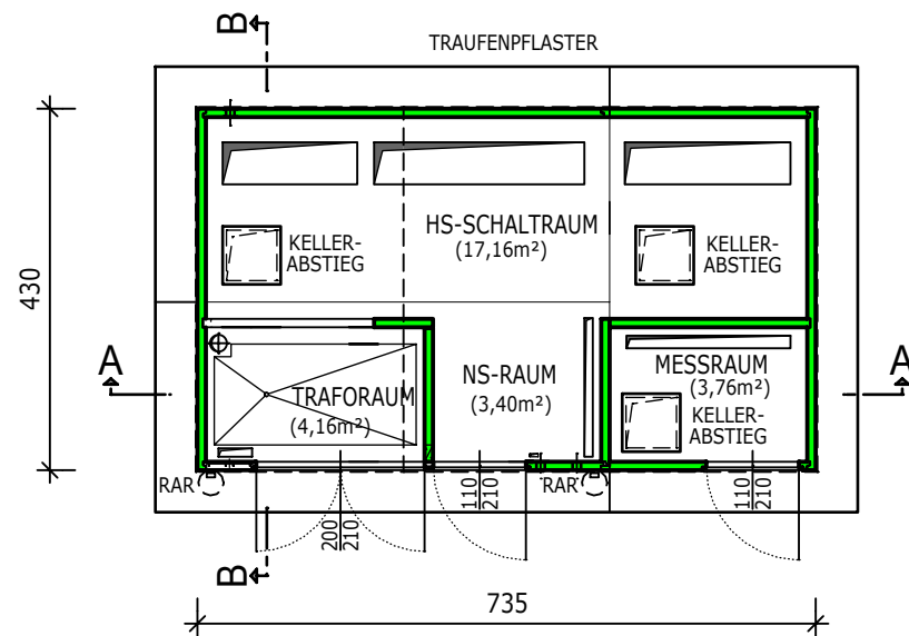
GRUNDRISS
