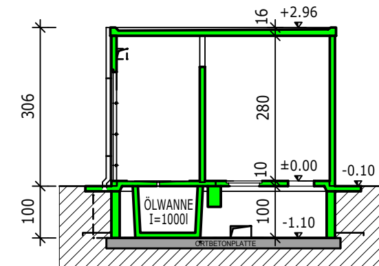
SCHNITT B-B
