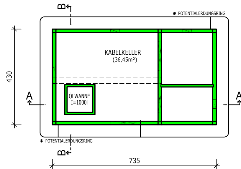
KABELKELLER
