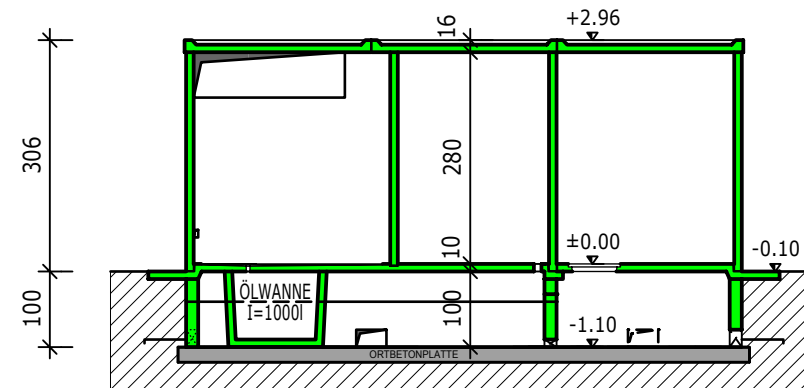
SCHNITT A-A
