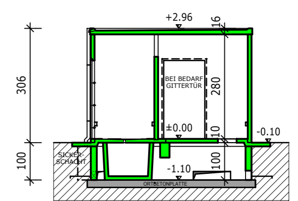
SCHNITT B-B
