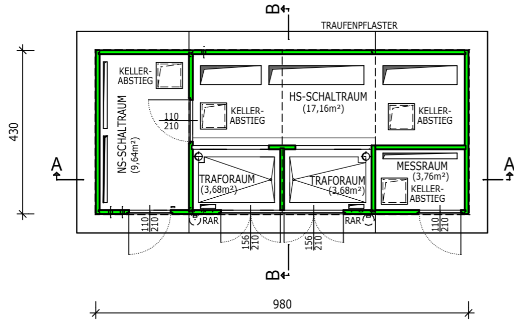
GRUNDRISS
