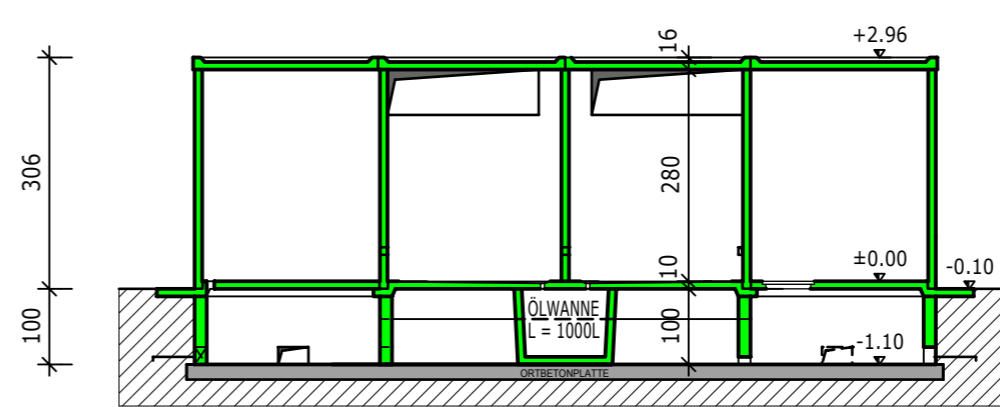
SCHNITT A-A
