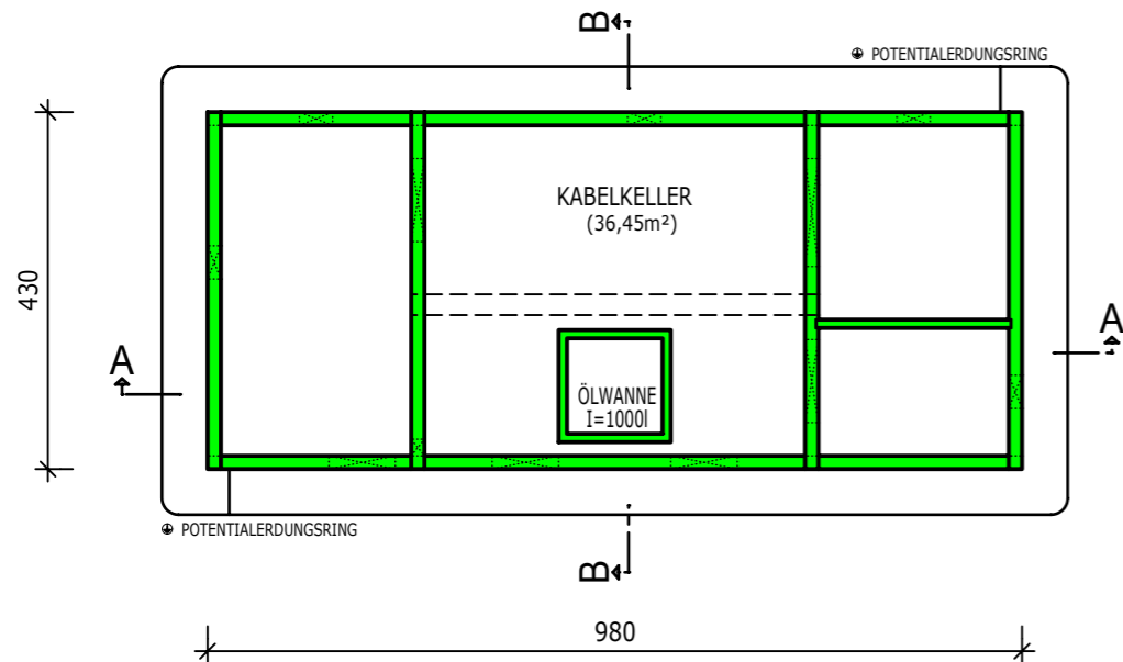
KABELKELLER
