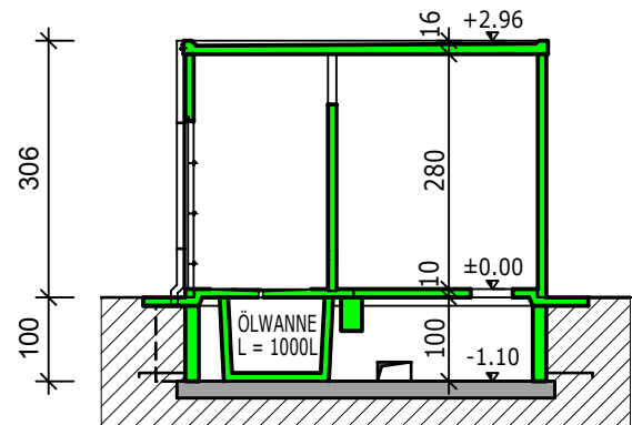
KABELKELLER
