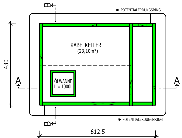
KABELKELLER
