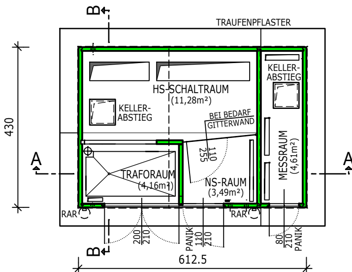
GRUNDRISS
