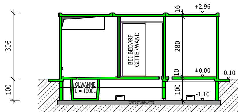
SCHNITT A-A
