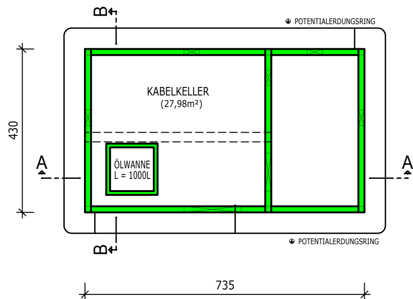
KABELKELLER
