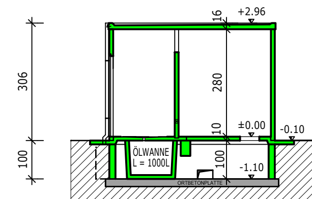
SCHNITT B-B
