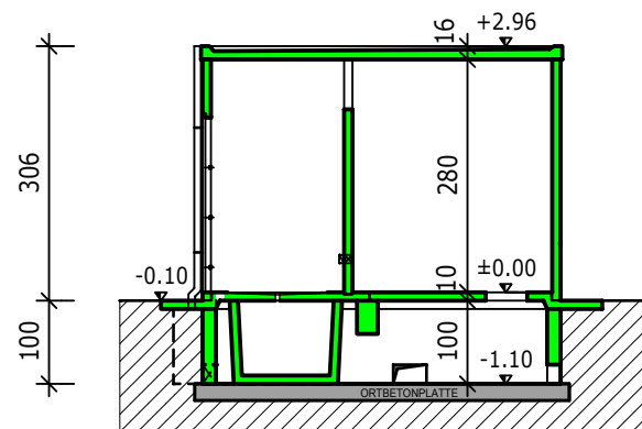
KABELKELLER
