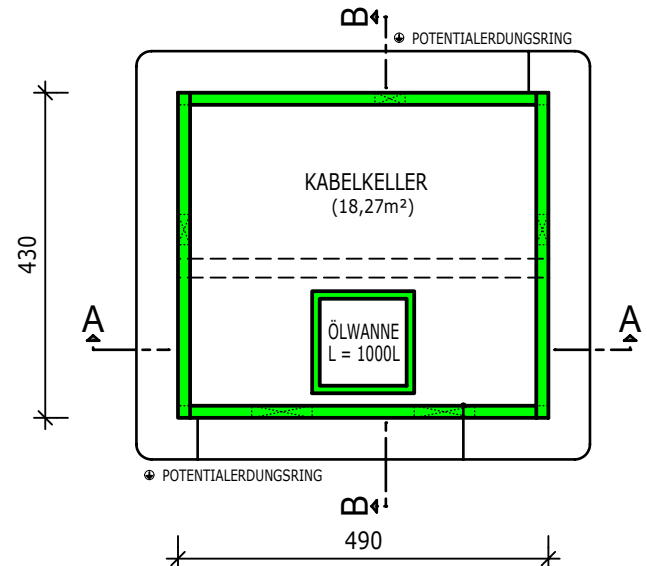
KABELKELLER
