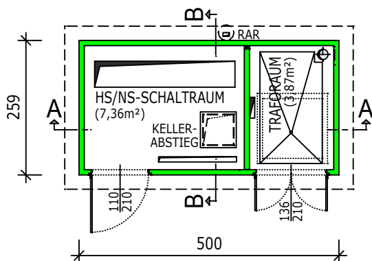
GRUNDRISS
