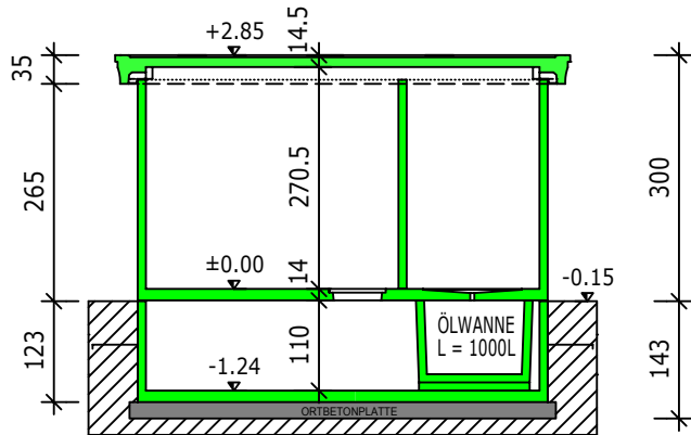
SCHNITT A-A
