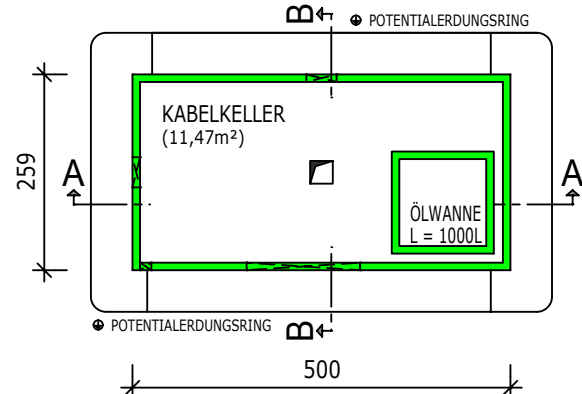
KABELKELLER
