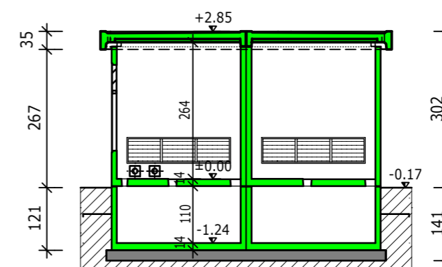
SCHNITT C-C
