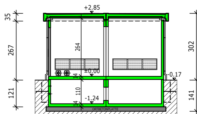
SCHNITT B-B
