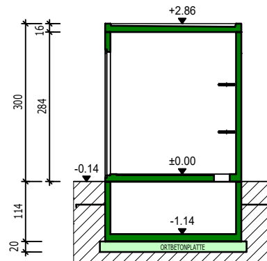
SCHNITT B - B
