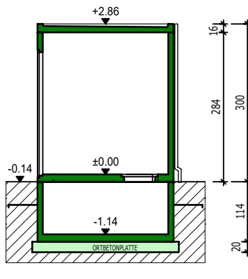
SCHNITT B - B
