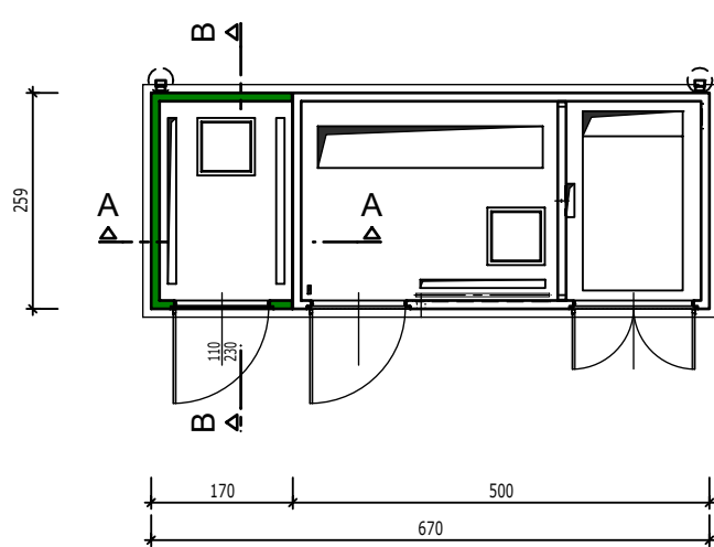
GRUNDRISS
