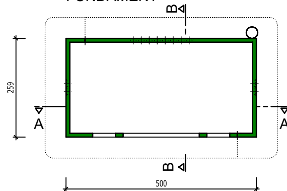
FUNDAMENT
